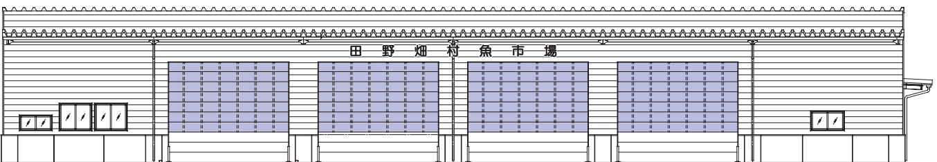
完成立面図
