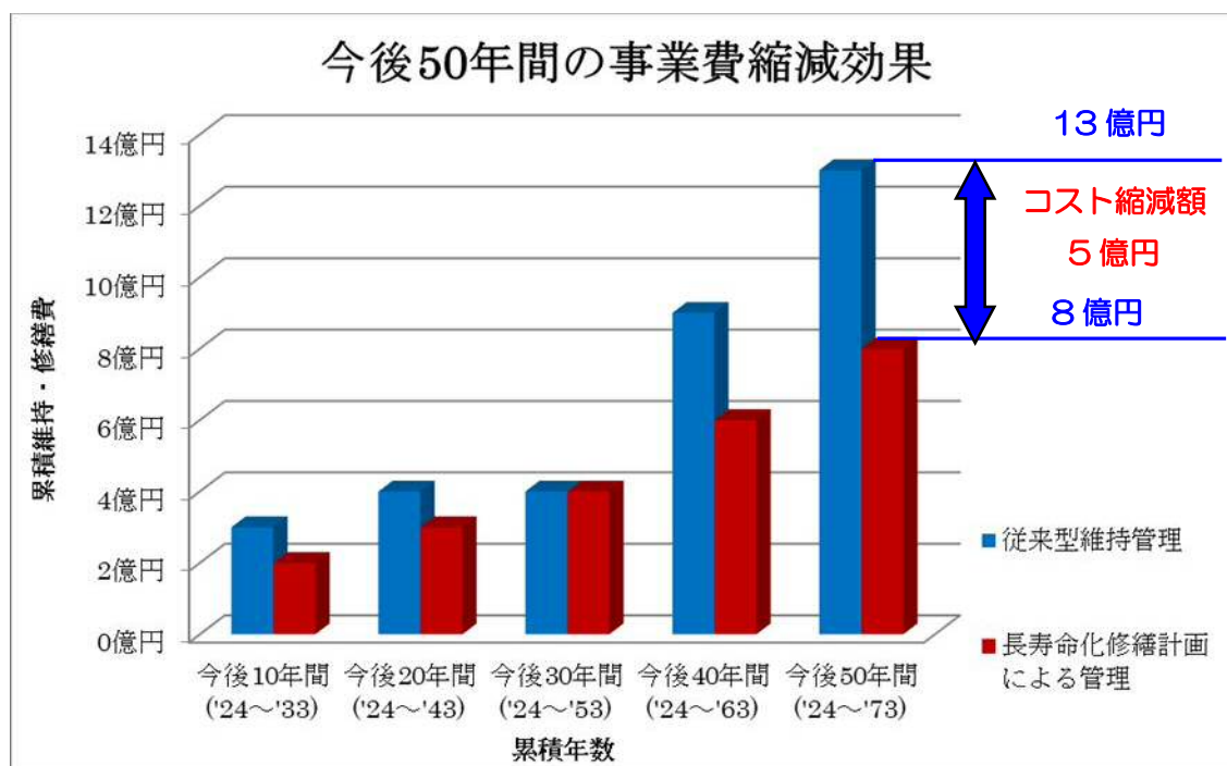
図-2 今後50年間における予防保全型と事後保全型の累積予算比較
